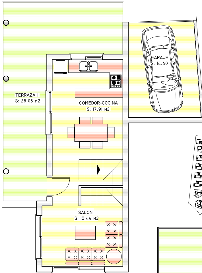
PLANTA BAJA
