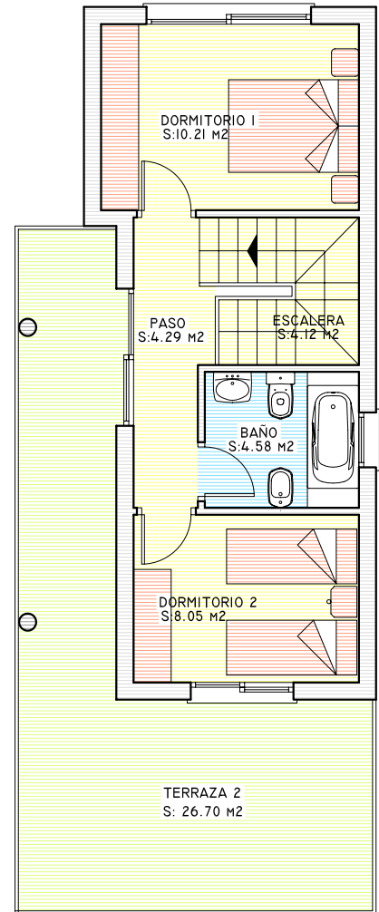
PLANTA SUPERIOR
